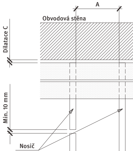
Obr. 2 Pokládka nosičů a vzdálenosti mezi nimi
